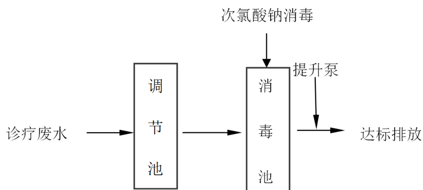
图 7 项目污水处理工艺流程图
