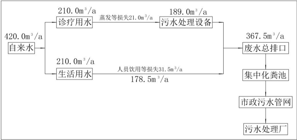
图 4 项目水平衡图
