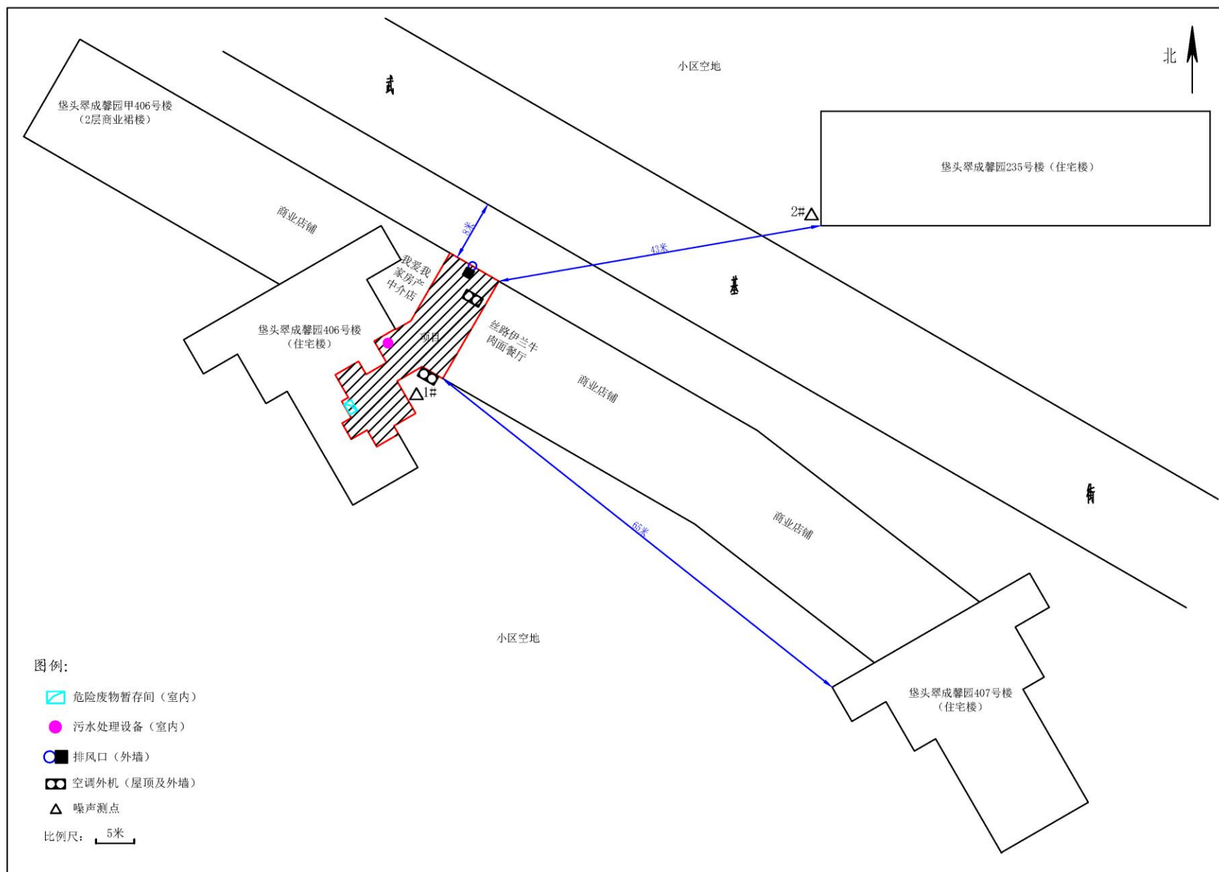
附图 2 建设项目周边关系及噪声测点图
