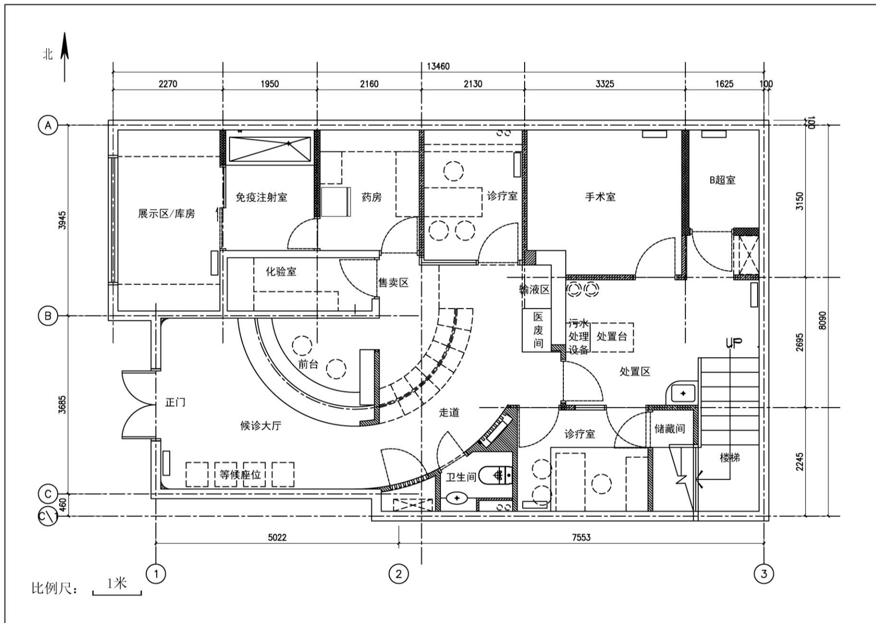
附图 3 建设项目一层平面布置图
