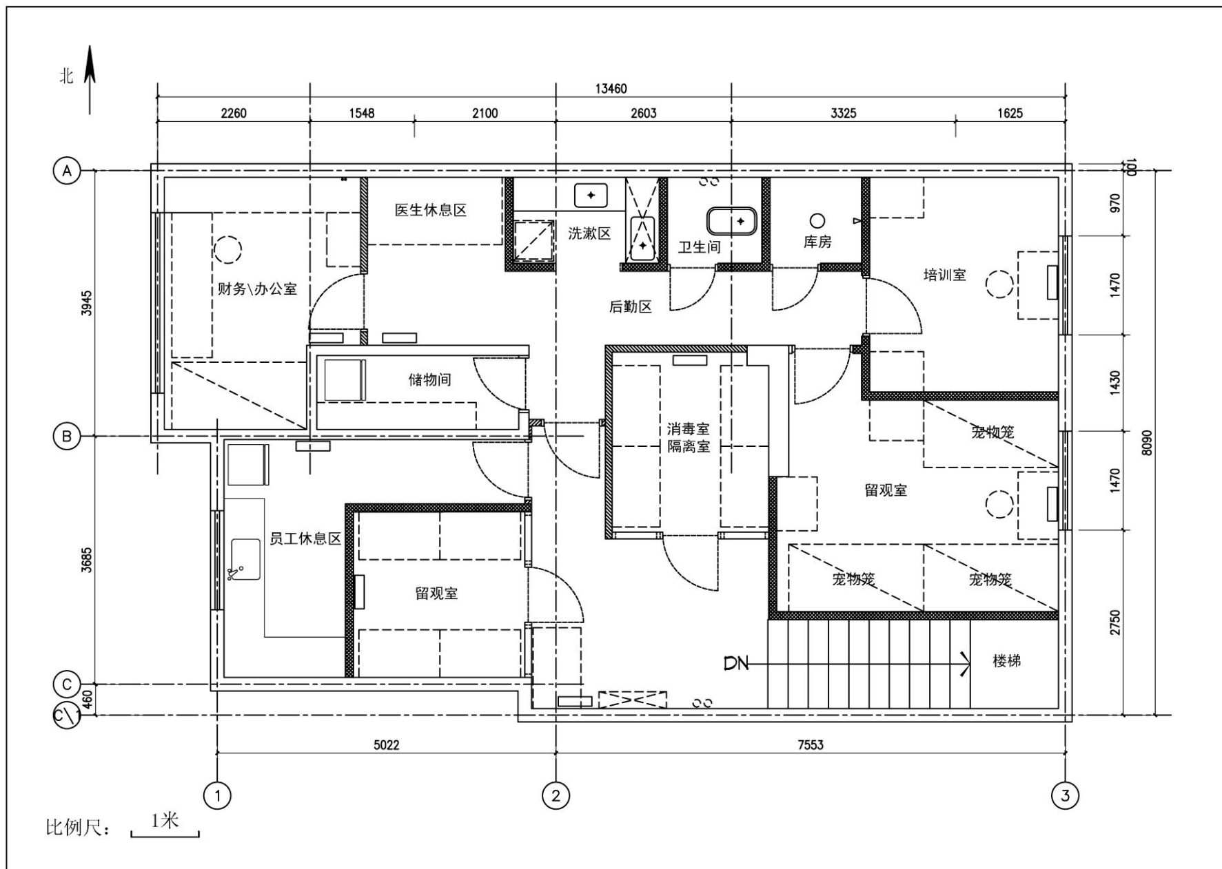
附图 4 建设项目二层平面布置图
