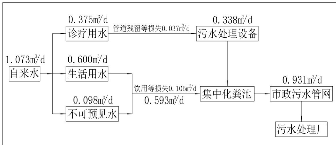
图 3 项目水平衡图
